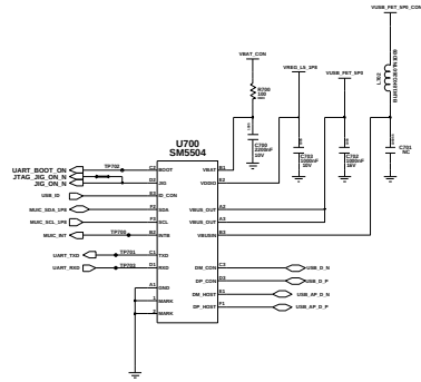
MUIC
